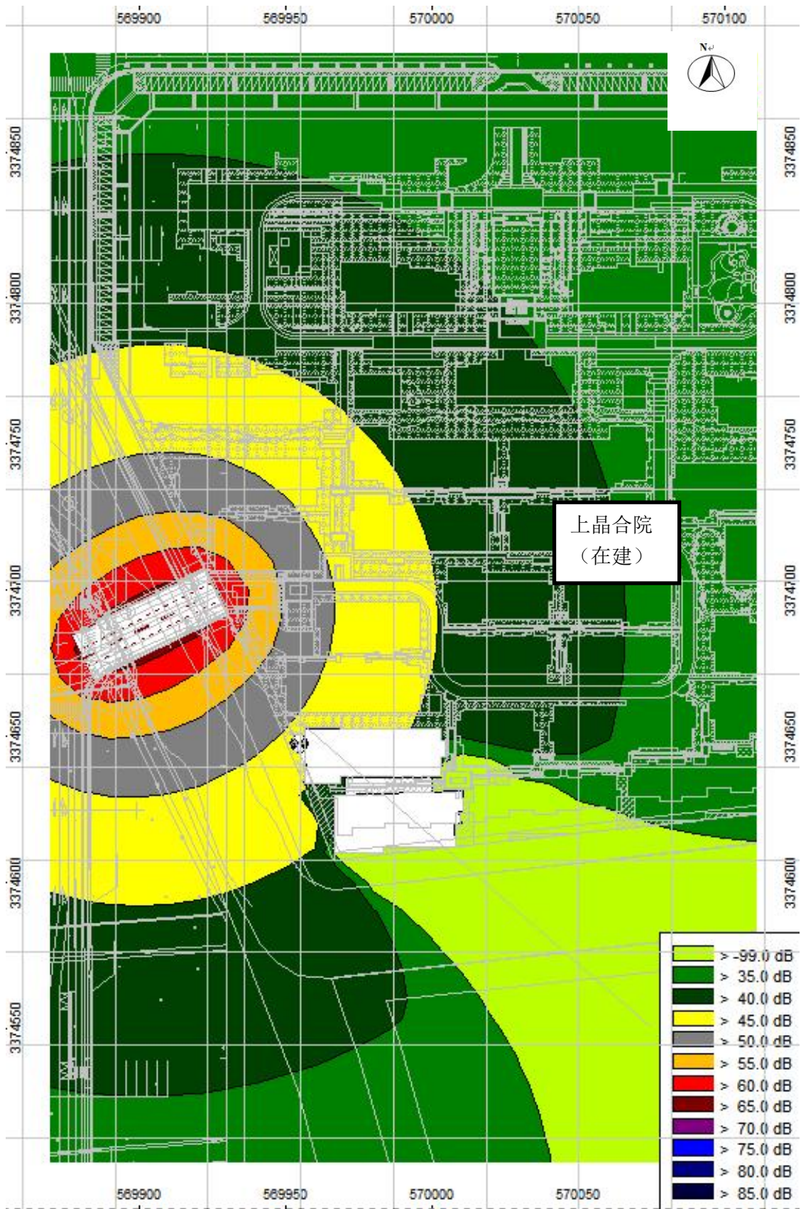
图 12 上品合院西侧桥梁典型路段夜间等声级线图（远期）
