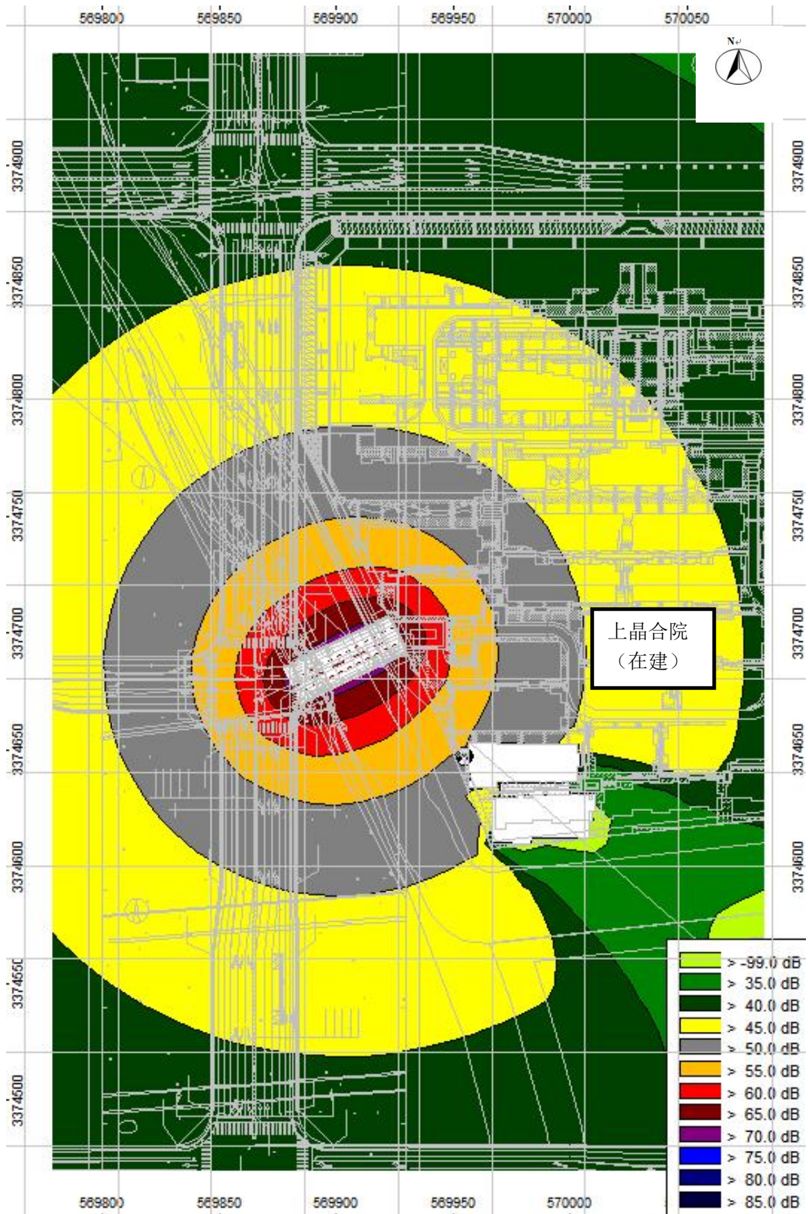
图9 上品合院西侧桥梁典型路段昼间等声级线图（中期）
