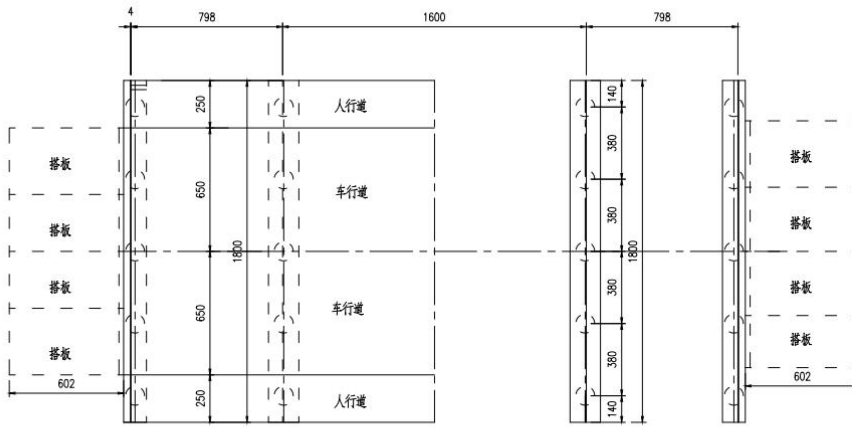
桥梁平面布置图
