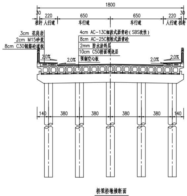
图 2-7 桥梁桥墩横断面图
