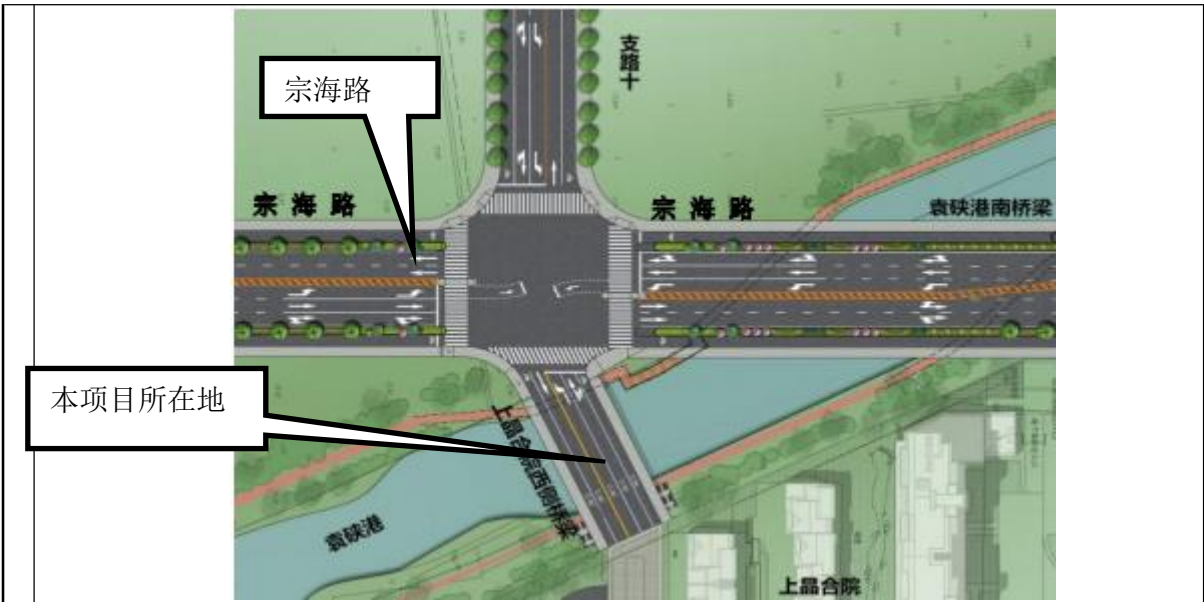
图 2-9 上晶合院西侧桥梁交叉口~宗海路交叉口交通组织
