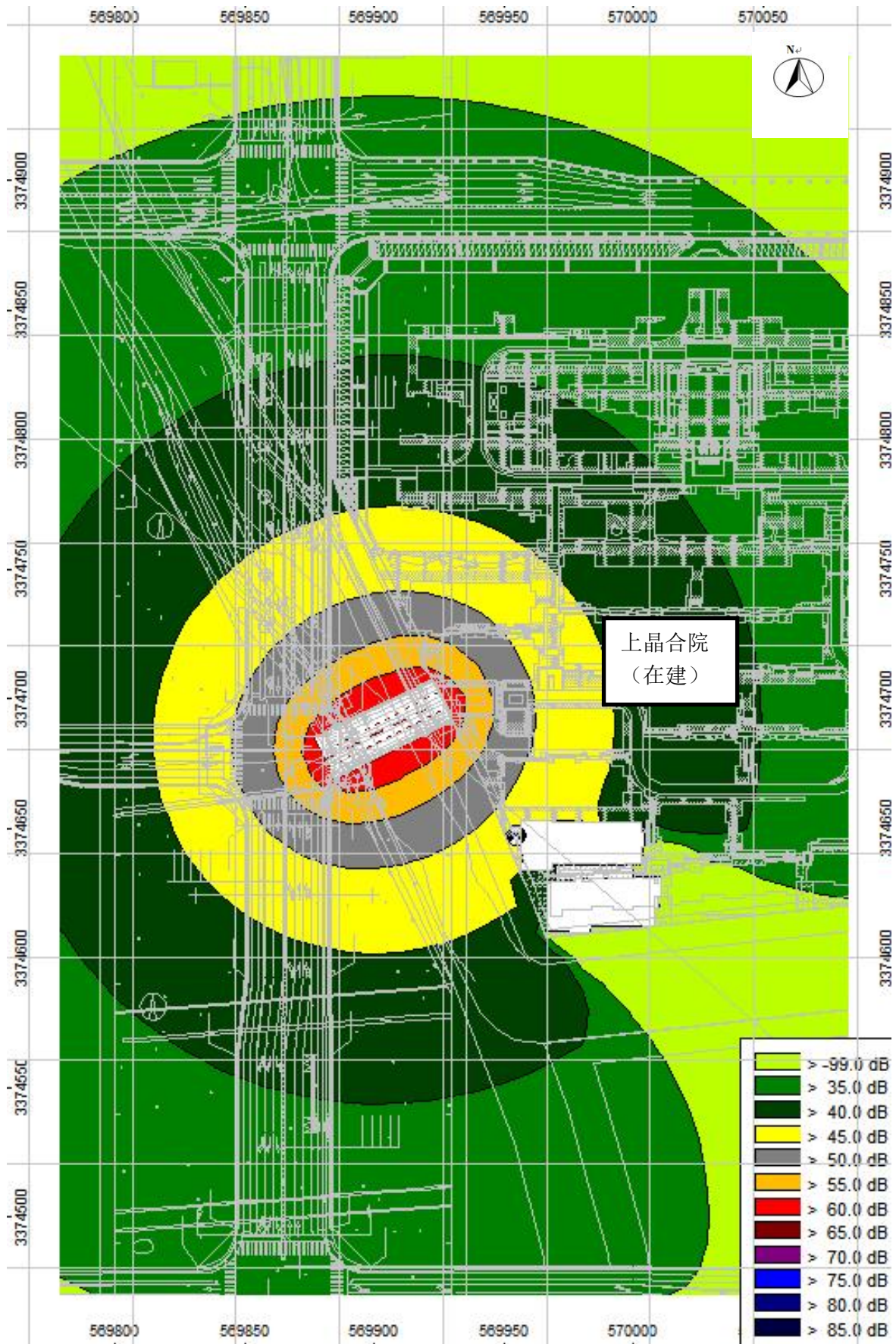
图 10 上晶合院西侧桥梁典型路段夜间等声级线图（中期）
