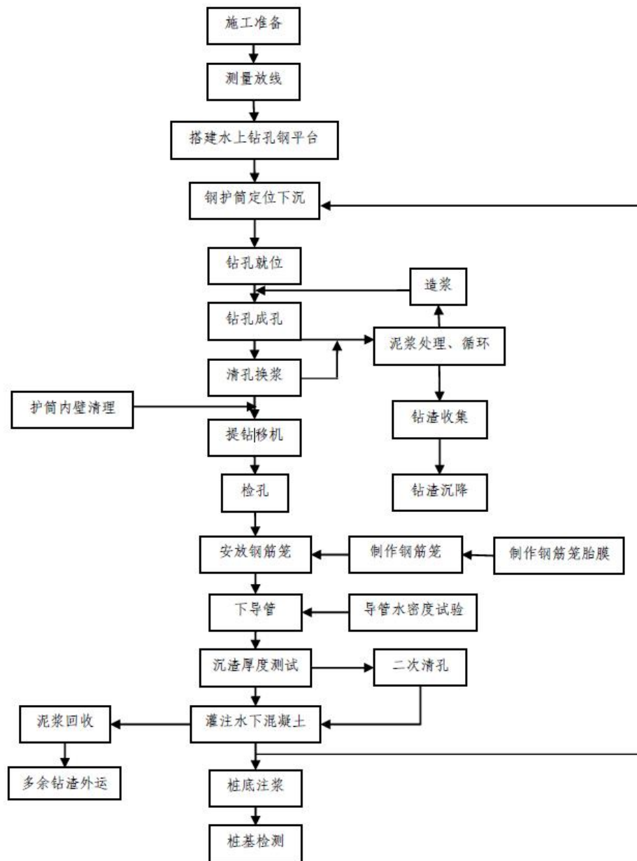
图2-13钻孔灌注桩施工工艺流程图
