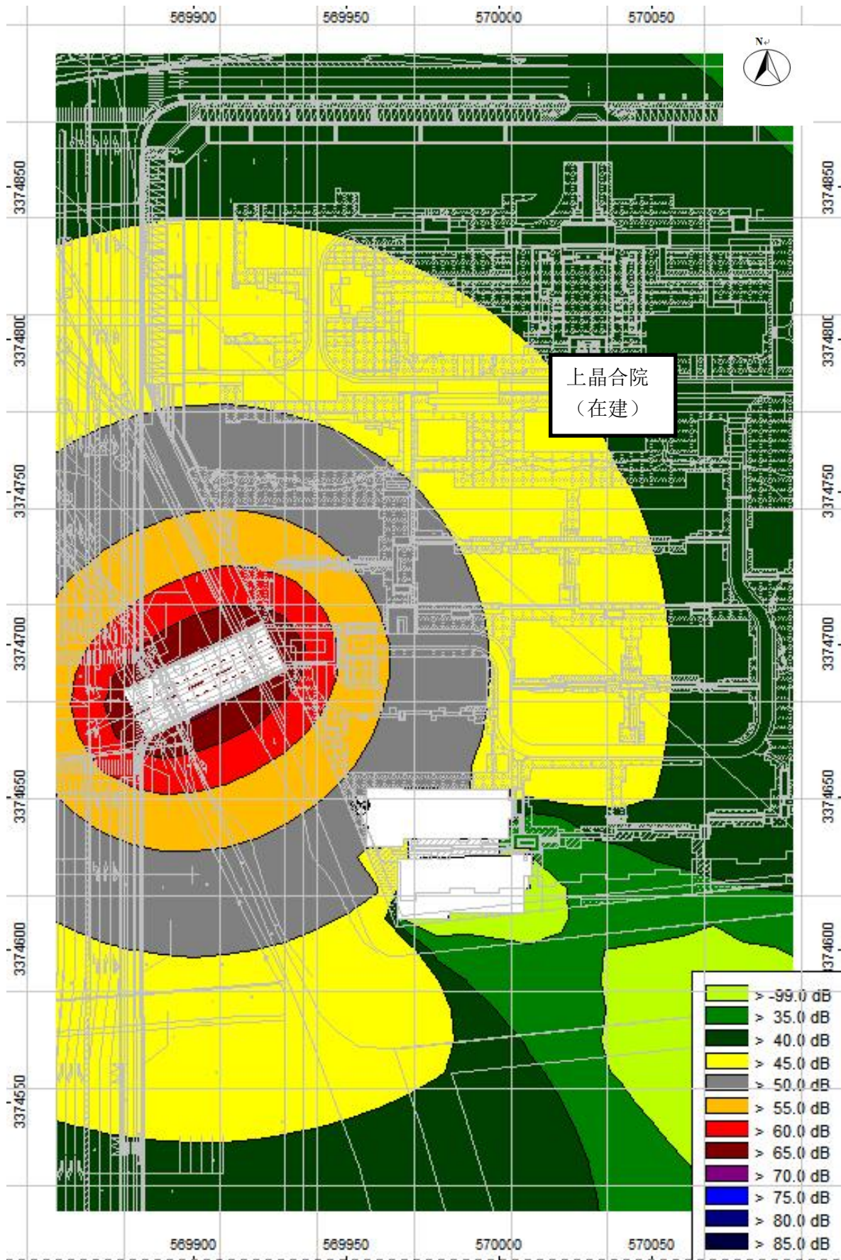
图 7 上品合院西侧桥梁典型路段昼间等声级线图（近期）
