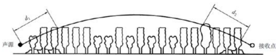
图 4 通过树和灌木时噪声衰减示意图
