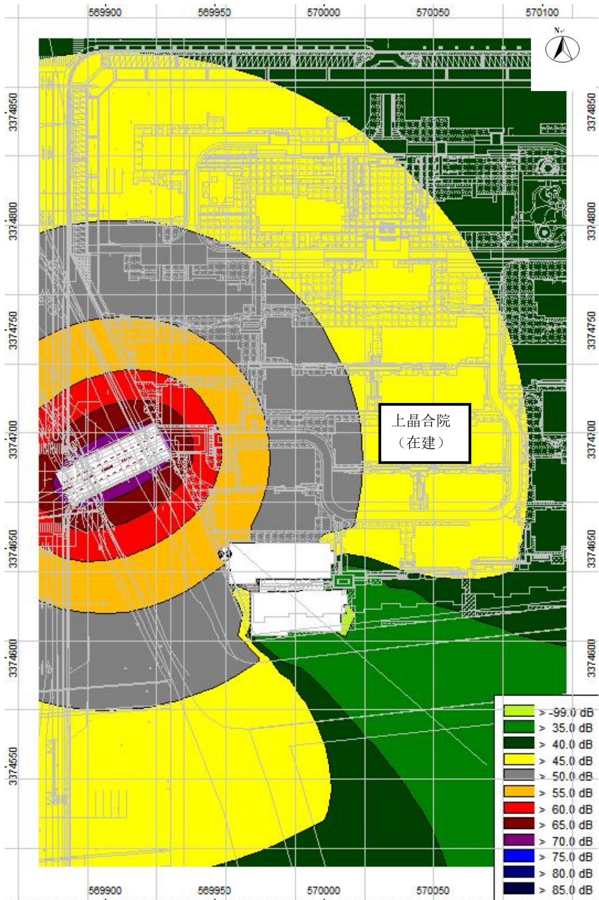
图 11 上品合院西侧桥梁典型路段昼间等声级线图（远期）
