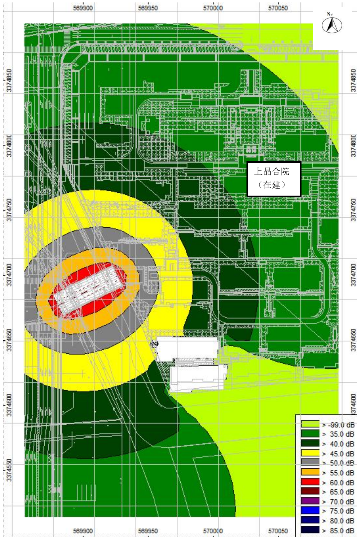
图 8 上品合院西侧桥梁典型路段夜间等声级线图（近期）
