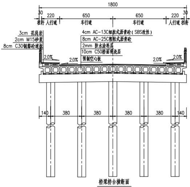
图 2-6 桥梁桥台横断面图
