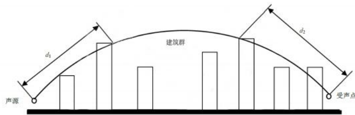
图 5 建筑群中声传播路径
