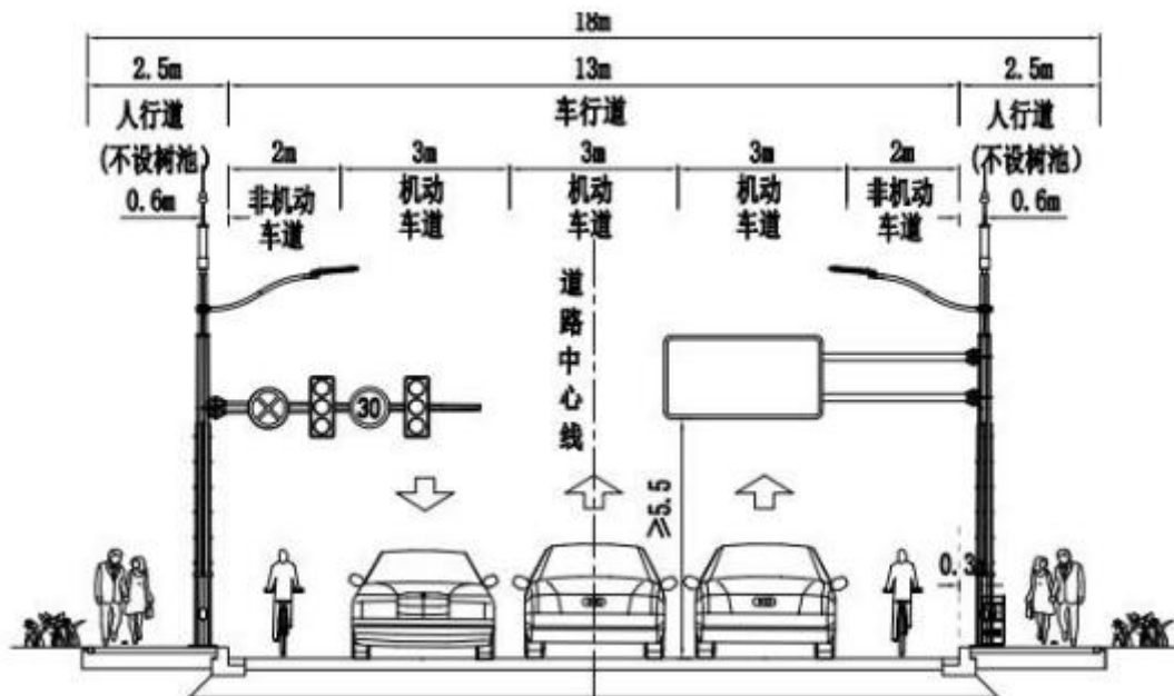
图 2-8 道路横断面图
