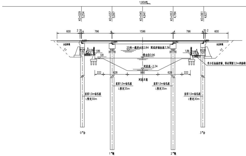
上晶合院西侧桥梁立面图 (8+16+8=32m)
