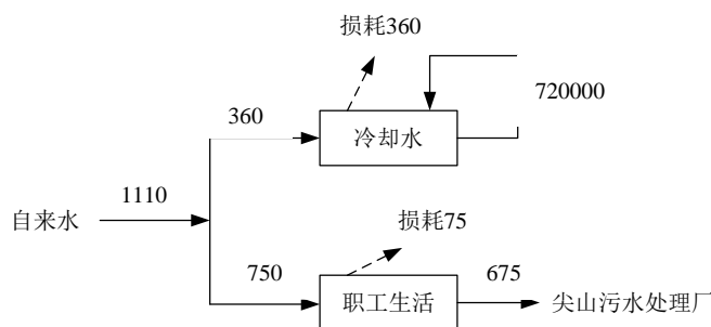
图2-1 本项目水平衡图
