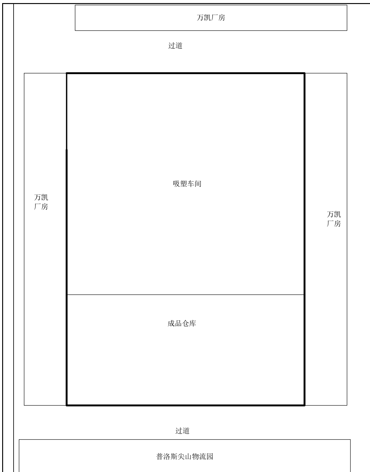
图4-6 企业三层土壤、地下水污染防治分区防渗图
