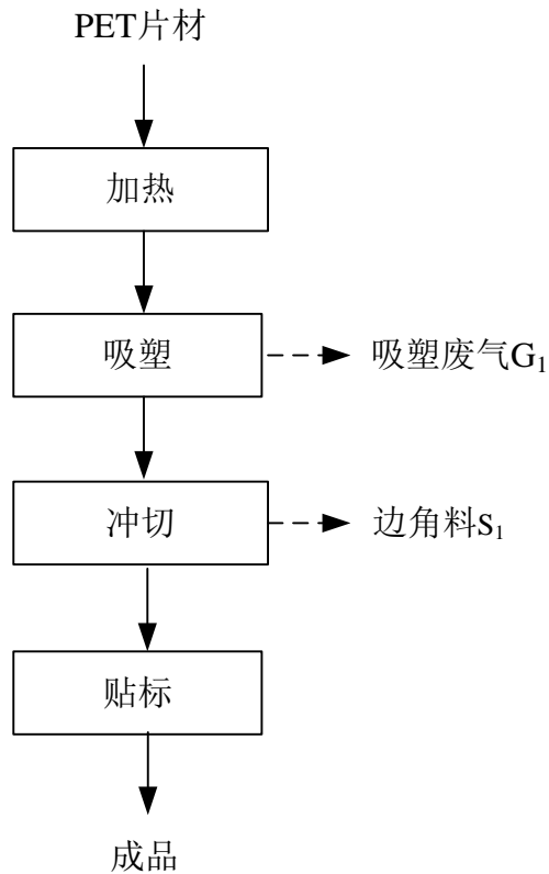
图2-1包装材料生产工艺
