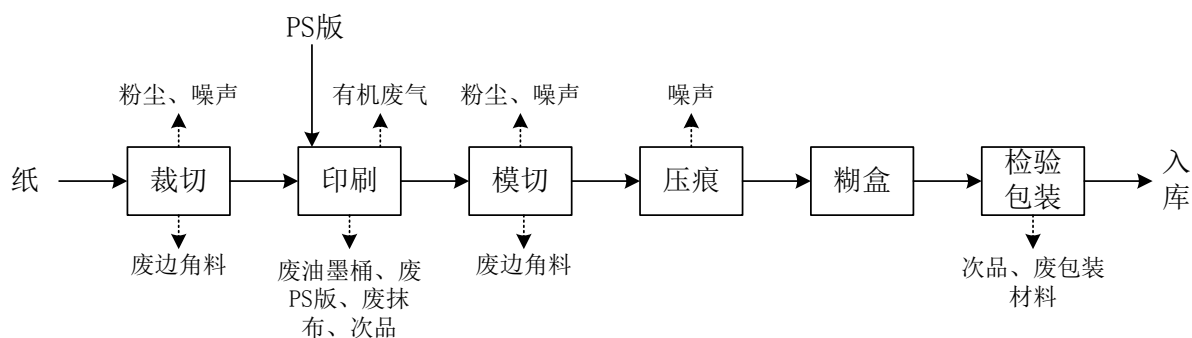
图 5-1 本项目印刷品的生产工艺流程及产污图
