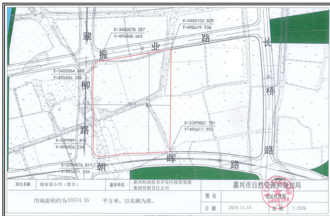
图 2.2-3 地块红线图
