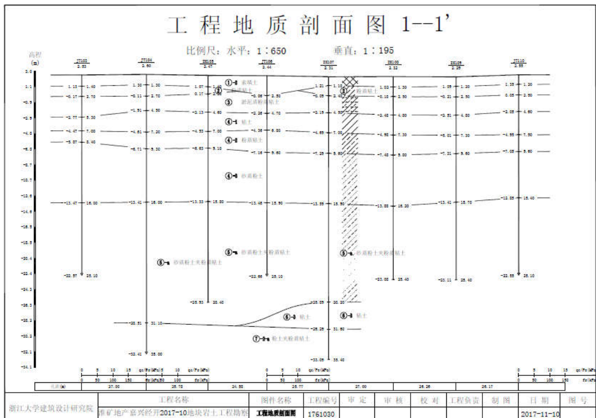
图 3.1-2 地质剖面图
